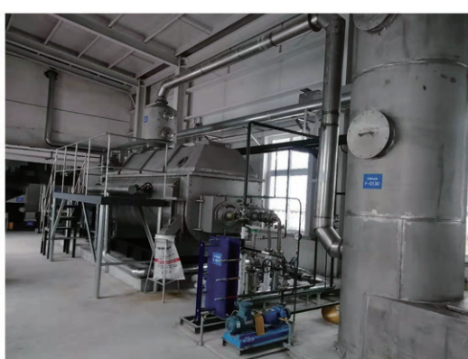
山东合生固废干燥现场
